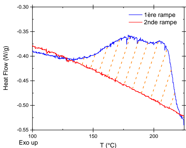
Figure II-4 : pic de décomposition des hydroperoxydes dans un EPDM réticulé au peroxyde
