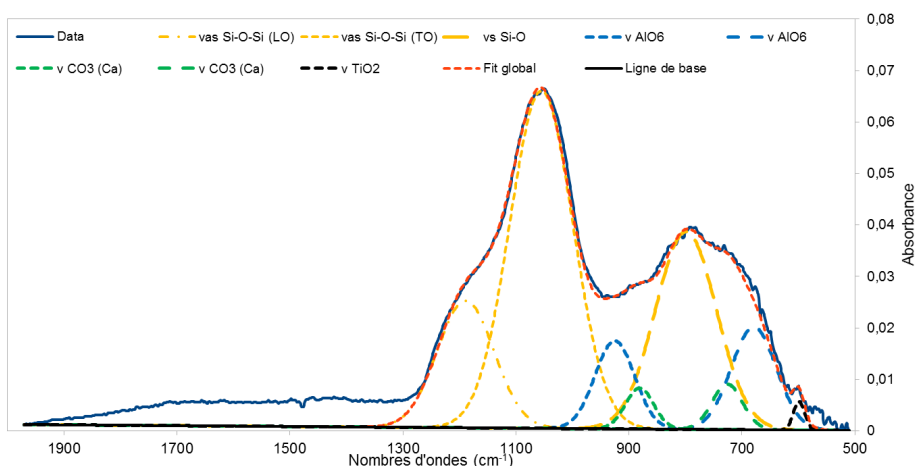
Figure V-18 : déconvolution sur la zone 500 cm -1 / 1900 cm -1 des résidus de pyrolyse sous O 2 à 600°C de l'EPDM A2
