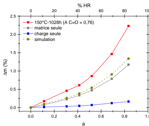
Figure V-133 : simulation de l'isotherme de sorption à 70°C de l'EPDM B1 préalablement vieilli 1028h à 150°C dans l'air en utilisant l'absorbance des carbonyles comme marqueur de vieillissement
