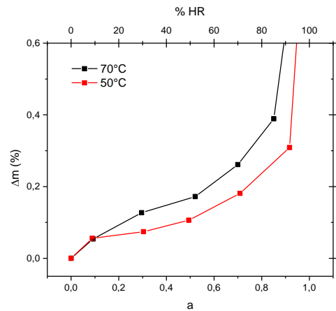
Figure V-95 : isotherme de sorption du matériau A2 à 50°C et 70°C sur tout l'intervalle (à gauche) et sur l'intervalle réduit [0,0,9] (à droite) d'activité en eau
