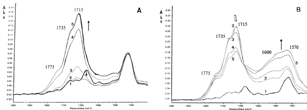
Figure I-33 : évolution du spectre ATR d'un EPDM chargé et réticulé au peroxyde au cours du vieillissement à 100°C dans l'air [A] 1 = 0h ; 2 = 3h30 ; 3 = 7h ; 4 = 21h ; 5 = 29h] ; [B] 1=0h ; 2 = 45h ; 3 = 88h ; 4 = 210h ; 5 = 395h] [31]
