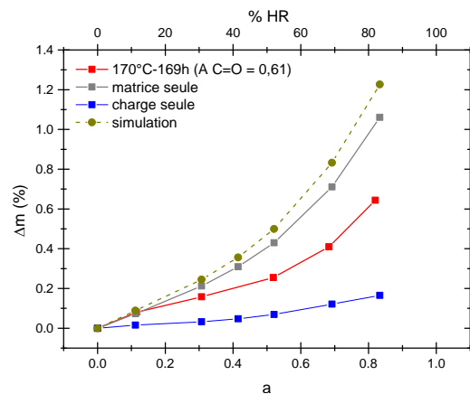
Figure V-131 : simulation de l'isotherme de sorption à 70°C de l'EPDM B1 préalablement vieilli 169h à 170°C dans l'air en utilisant l'absorbance des carbonyles comme marqueur de vieillissement
