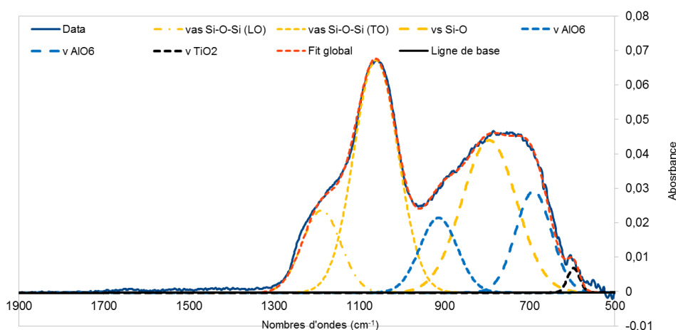
Figure V-19 : déconvolution sur la zone 500 cm -1 / 1900 cm -1 des résidus de pyrolyse sous O 2 à 600°C de l'EPDM A4
