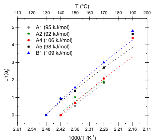
Figure V-94 : courbes d'Arrhenius obtenues pour le facteur de translation en temps pour la T_g pour le matériau A1 (hexagone gris), A2 (étoile jaune foncée), A4 (rond rouge), A5 (carré noir) et B1 (triangle bleu)
