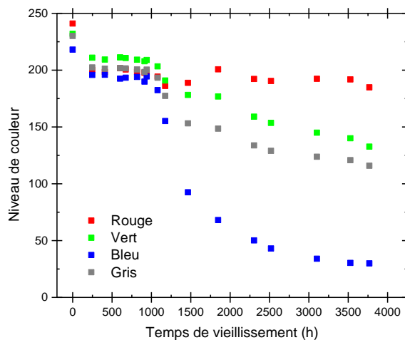
Figure V-27 : évolution des différentes teintes avec le temps de vieillissement dans l'air à 90°C pour l'EPDM C
