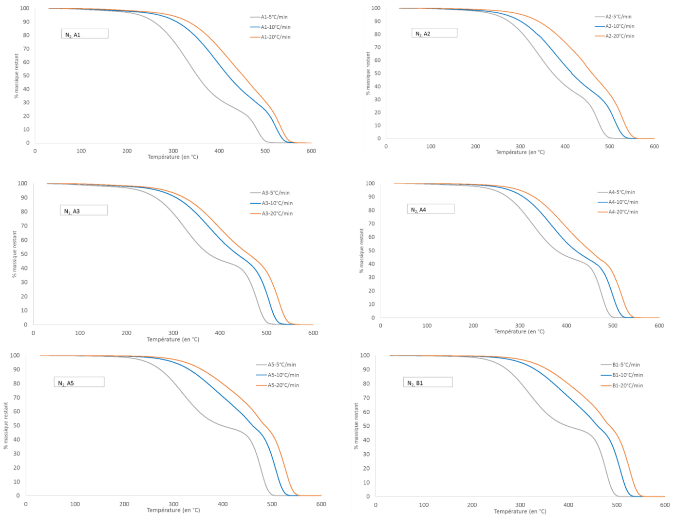
Figure V-16 : ensemble des courbes étalonnées sous atmosphère 100% N 2 à 5°C/min, 10°C/min et 20°C/min.
