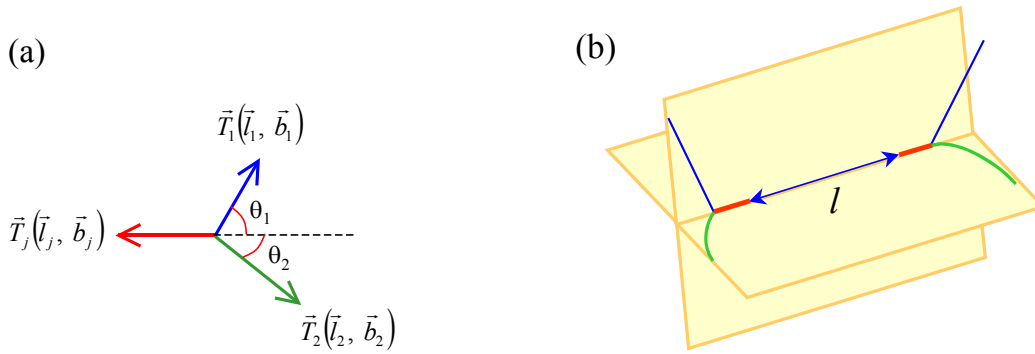
Fig. 20: (a) équilibre sur un nœud triple et (b) dislocation ancrée sous contrainte.
