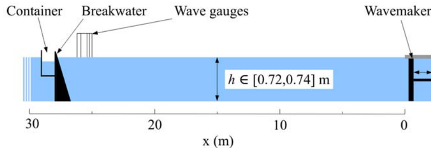
Figure 2. Schéma indicatif du canal-soufflerie de l'OSU Pythéas indiquant la position de la digue et des instruments de mesure. Une unité verticale vaut 5 unités horizontales.
