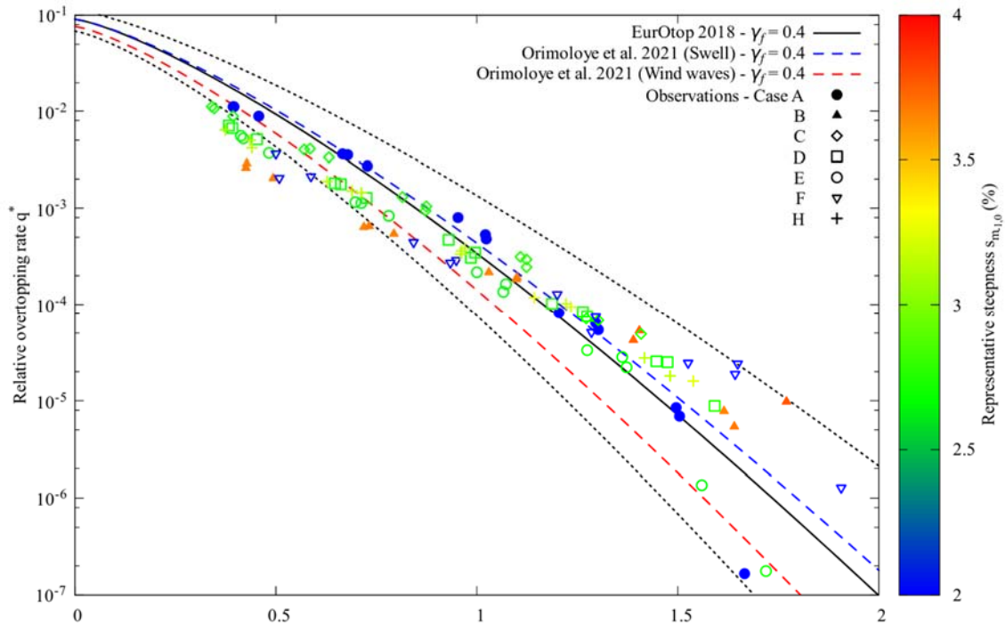
Figure 5. Débit de franchissement adimensionnel en fonction de la hauteur de franc-bord adimensionnelle de la digue avec enrochements. Chaque point correspond au résultat d'un essai de 30 min. Les points sont colorés par la cambrure représentative de l'état de mer. Un coefficient de rugosité \gamma_f = 0.4 est appliqué dans l'équation (6) pour les courbes EurOtop (2018) et ORIMOLOYE et al. (2021). La courbe en pointillés noir représente l'intervalle de confiance à un niveau de précision de 90 %.
